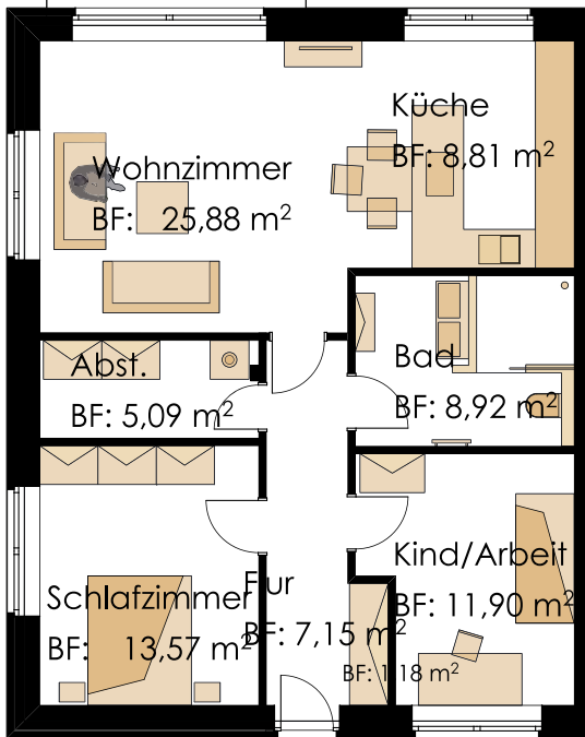
Beispielhafter Grundriss
